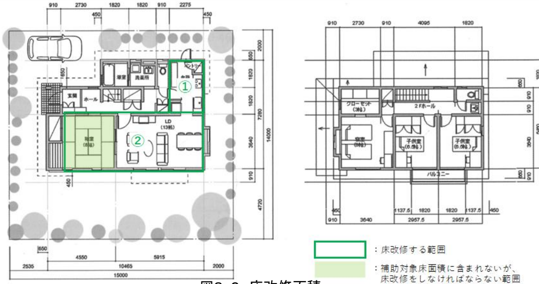
図8-2 床改修面積
