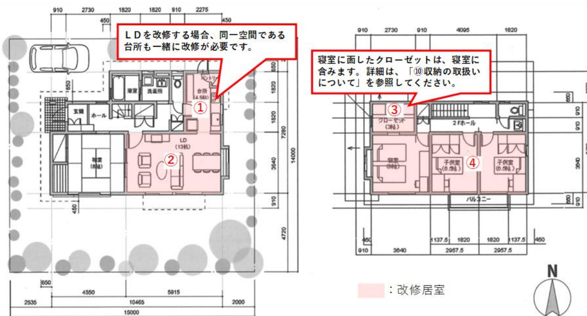
図4-2 改修面積算定
