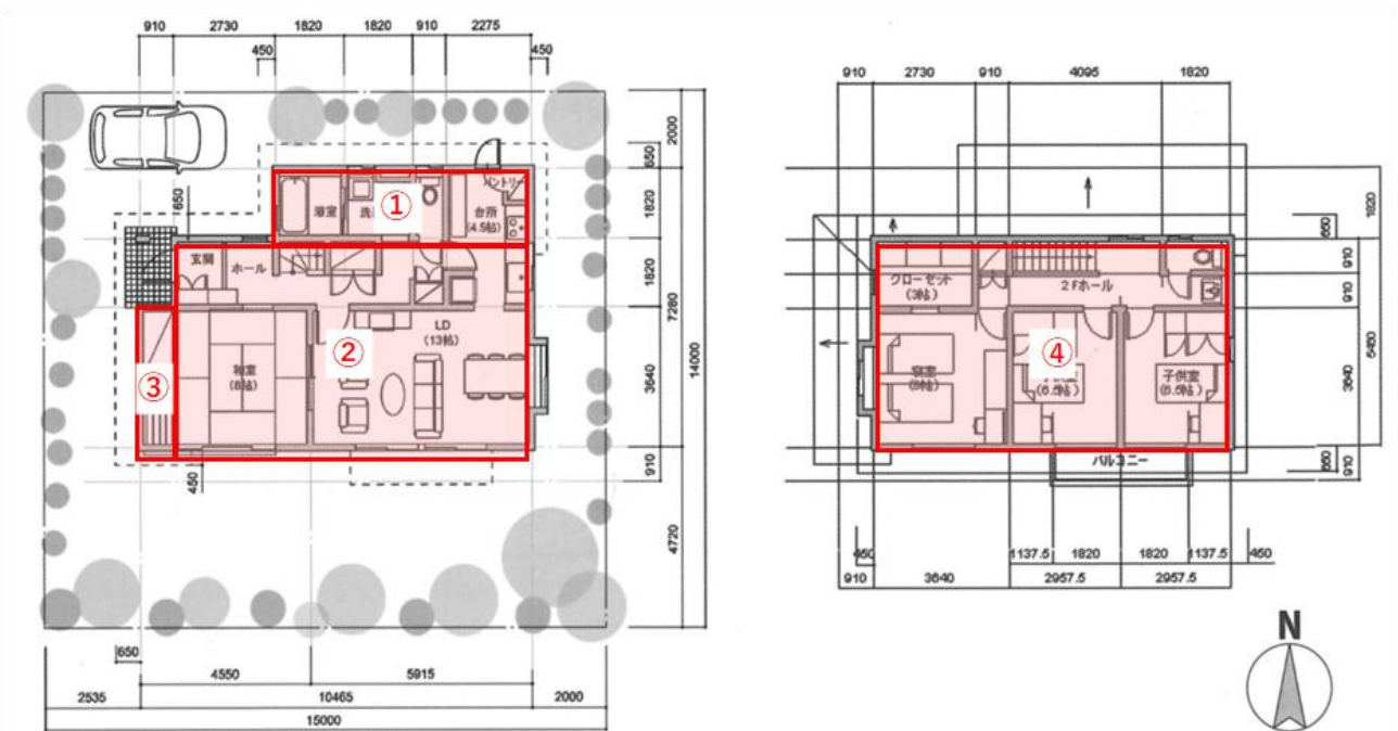
図3 延べ床面積算定
