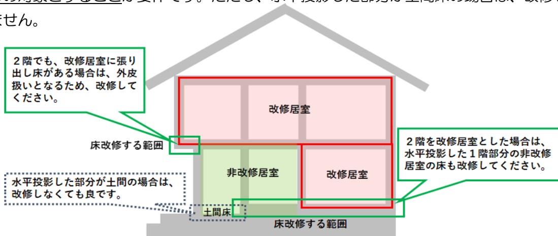
図8-1 床断熱改修
