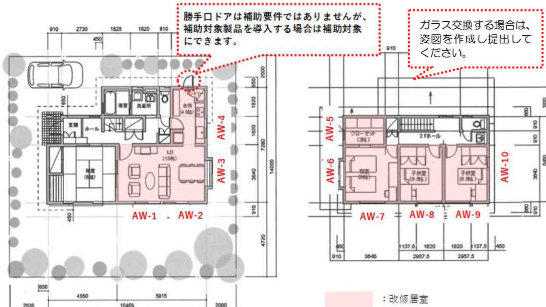
図9 窓改修寸法
