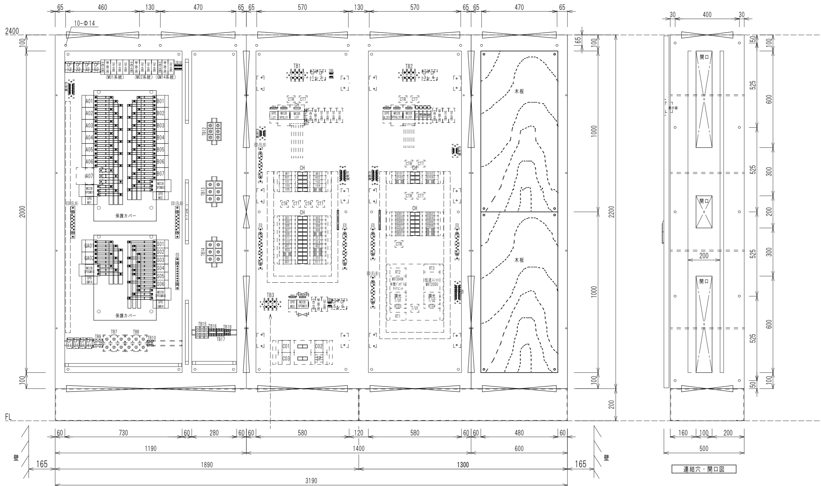
内面図
