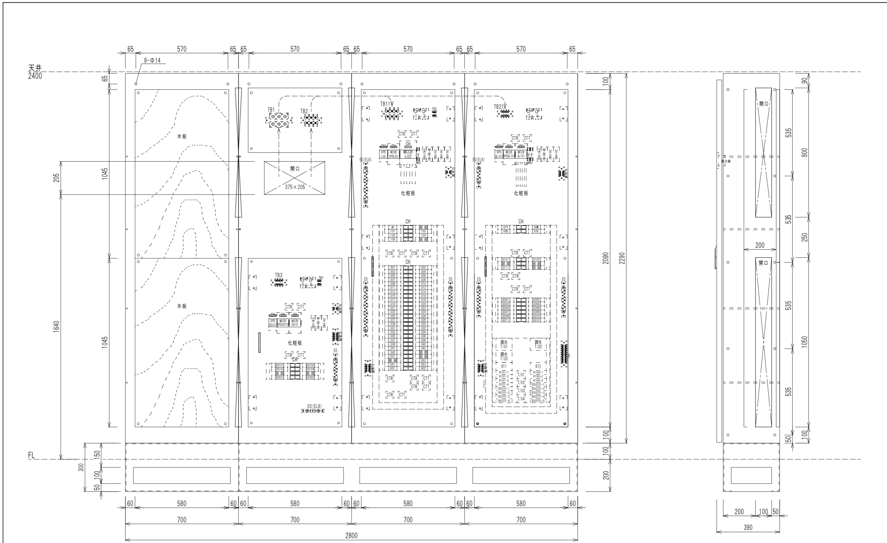
内面図
