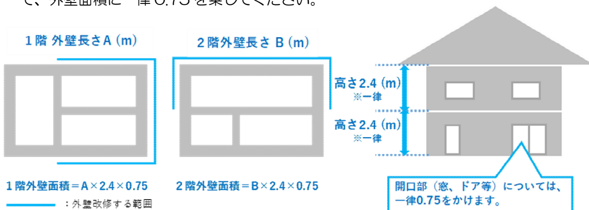
図7-1 外壁断熱改修
