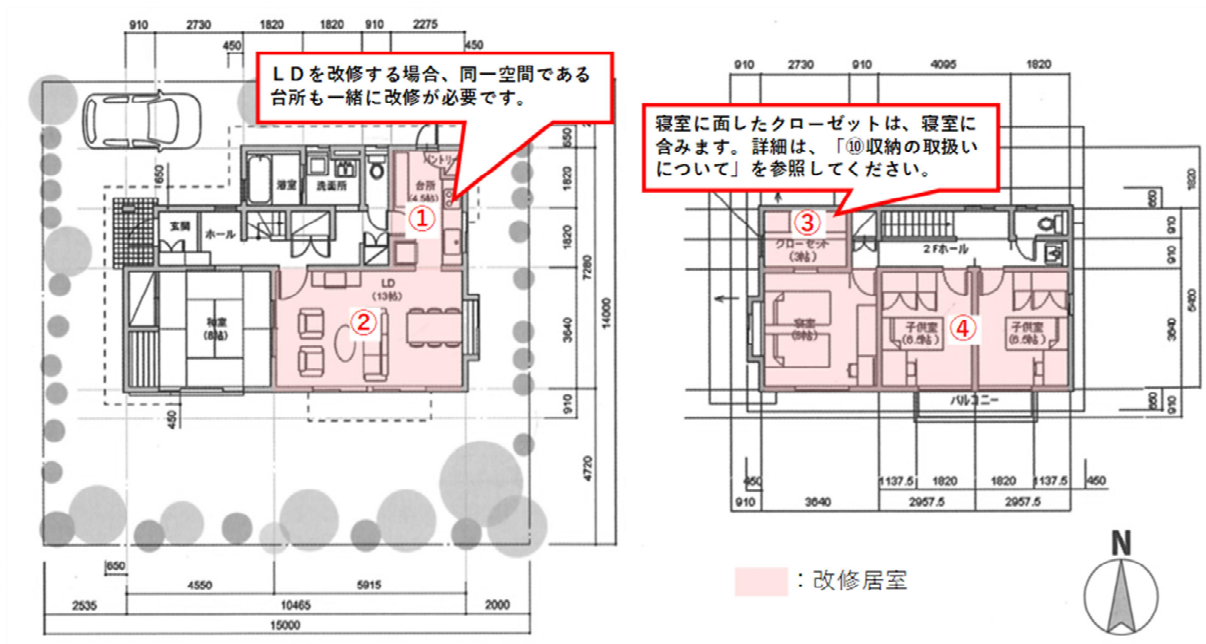
図4-2 改修面積算定
